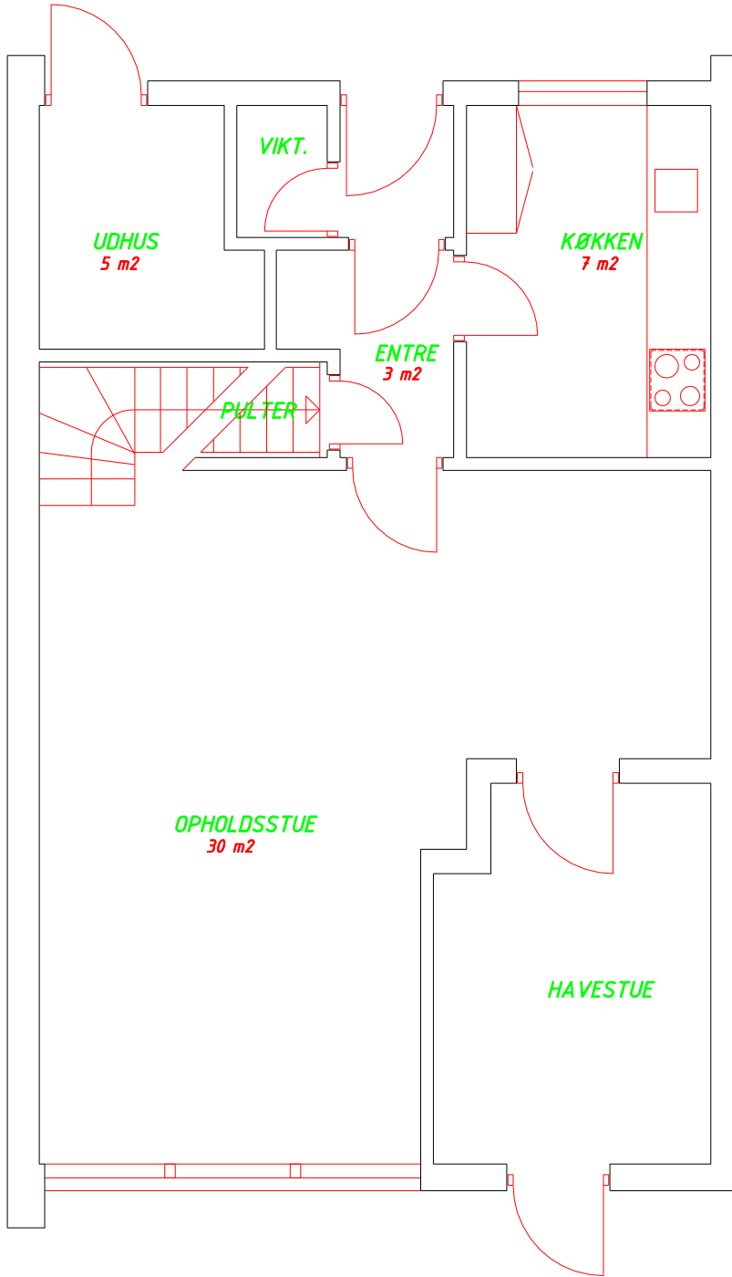
STUEPLAN
