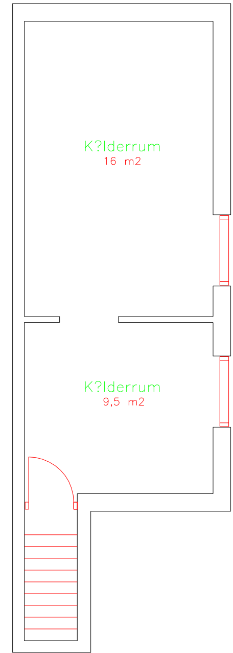
KÆLDERPLAN
